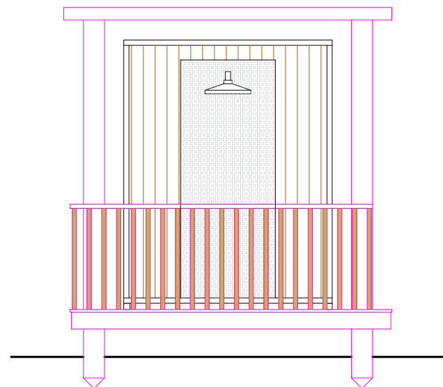
Modulo Prospetto laterale con pergola
