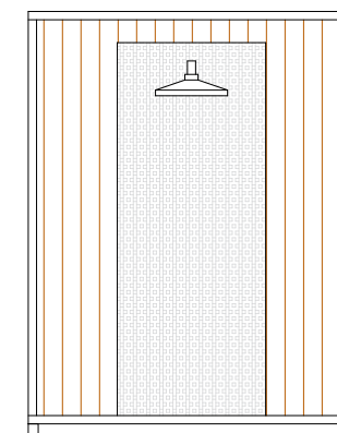
Modulo Prospetto Laterale
