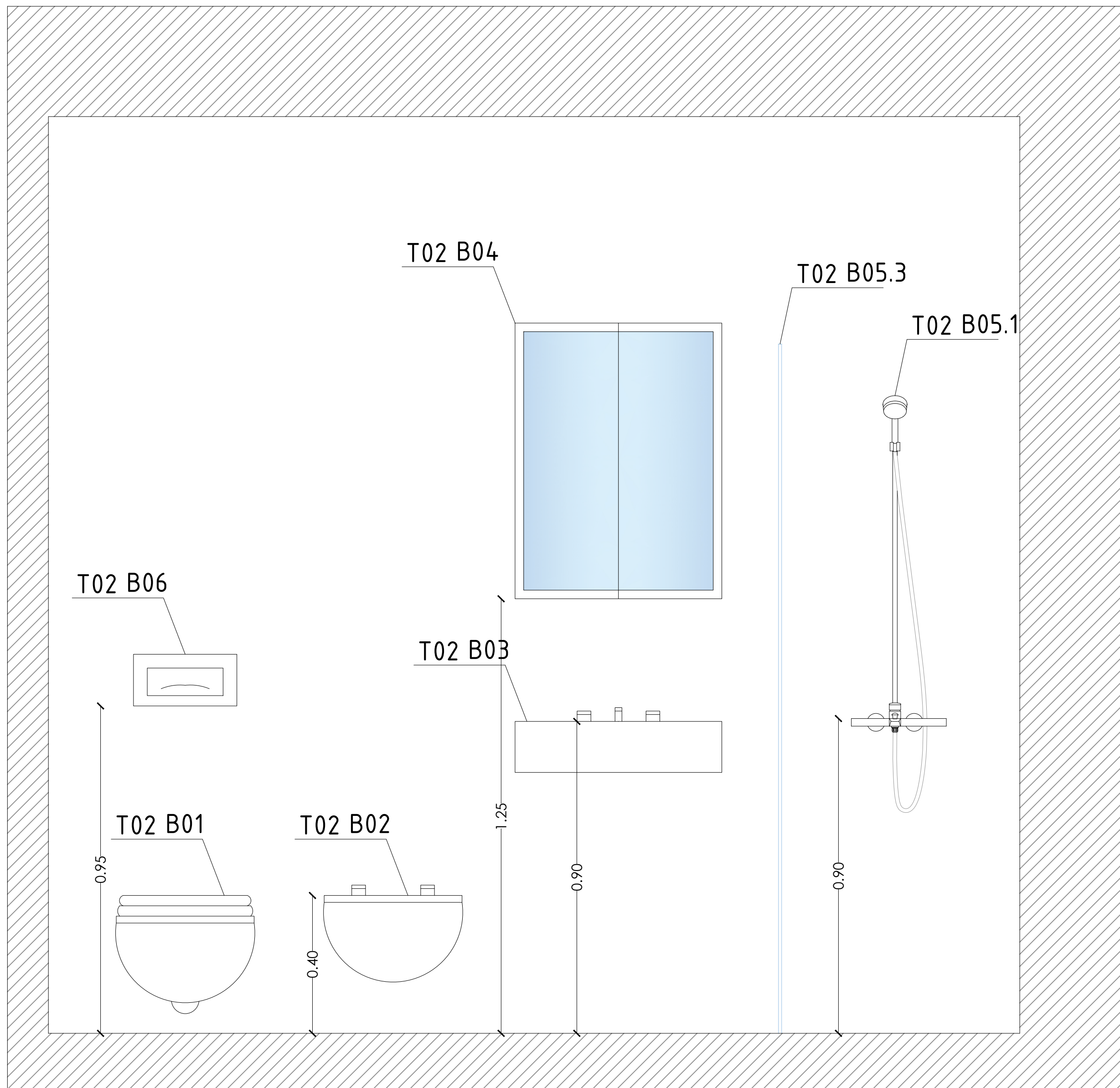
BAGNO - PROSPETTO 4
