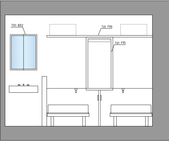
CAMERA TIPO - PROSPETTO 1
