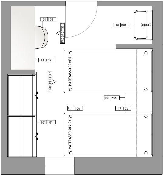
CAMERA TIPO - PLANIMETRIA ARREDATA
