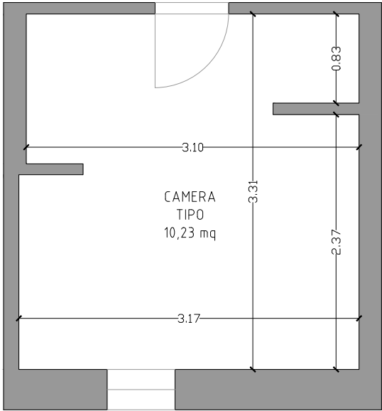
CAMERA TIPO - PLANIMETRIA QUOTATA
