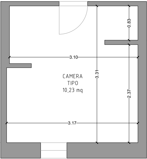
CAMERA TIPO - PLANIMETRIA QUOTATA
