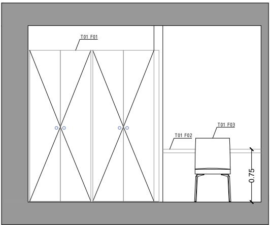
CAMERA TIPO - PROSPETTO 2
