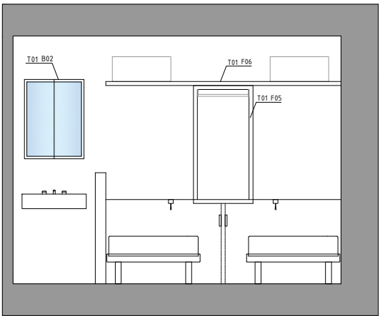
CAMERA TIPO - PROSPETTO 1
