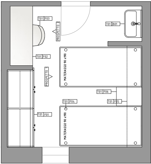
CAMERA TIPO - PLANIMETRIA ARREDATA
