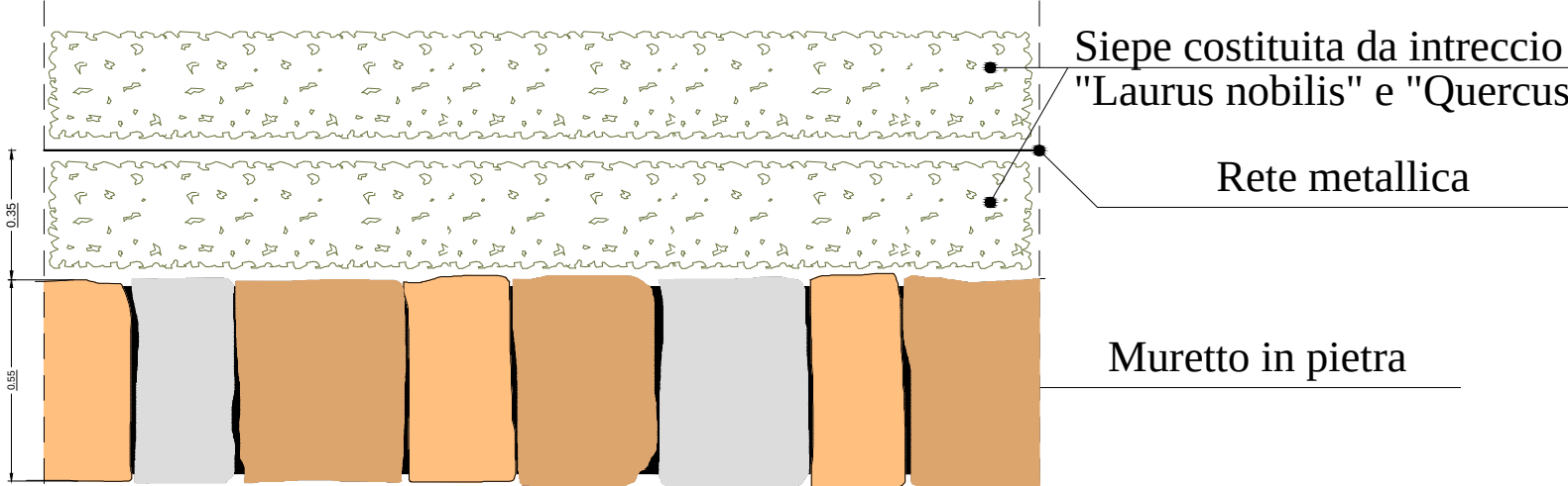
Particolare Pianta scala 1:20
