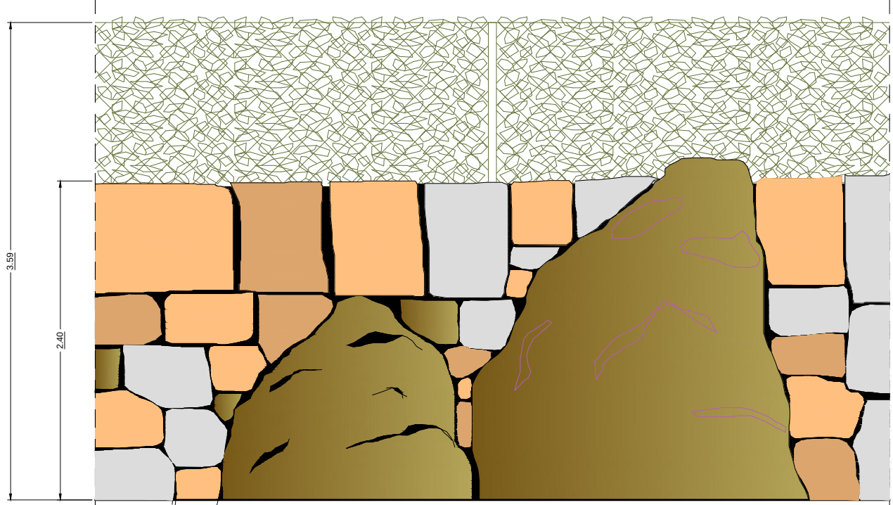
Particolare Prospetto Vista dalla Strada scala 1:20
