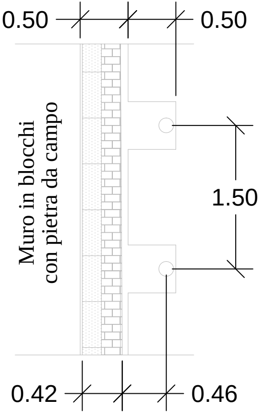
Pianta schema fondazione e pali
