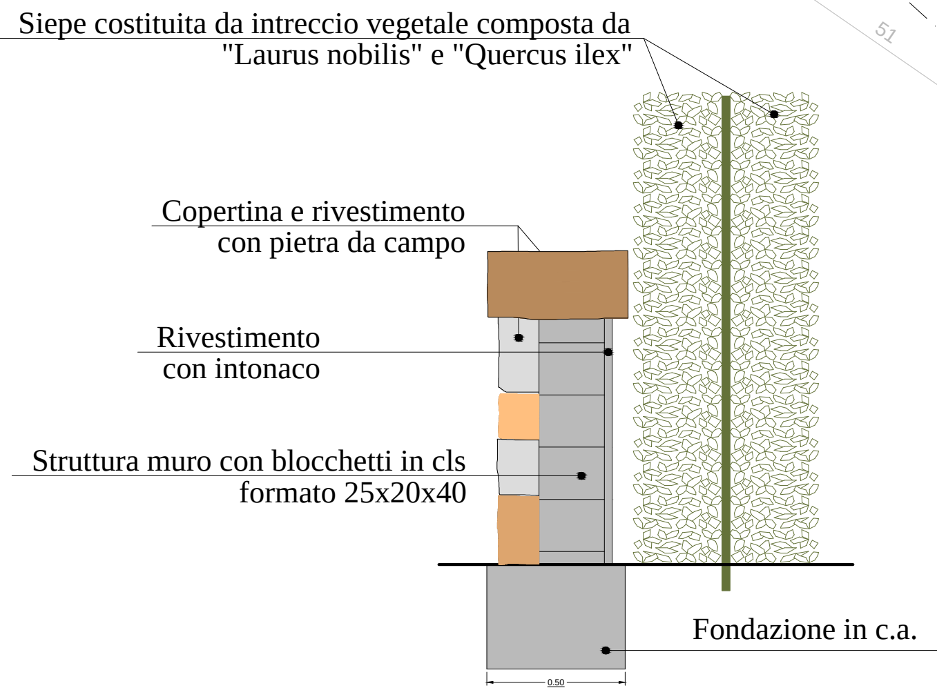
Sezione Tipo scala 1:20
